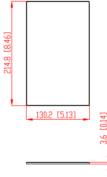
TRIMLESS GRILLE
